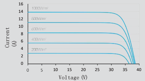
Power-Voltage (425W)
